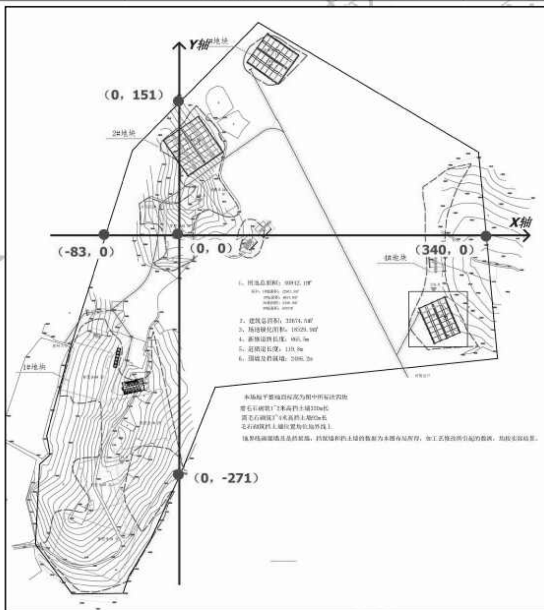
图 5-9 声环境预测坐标体系图
