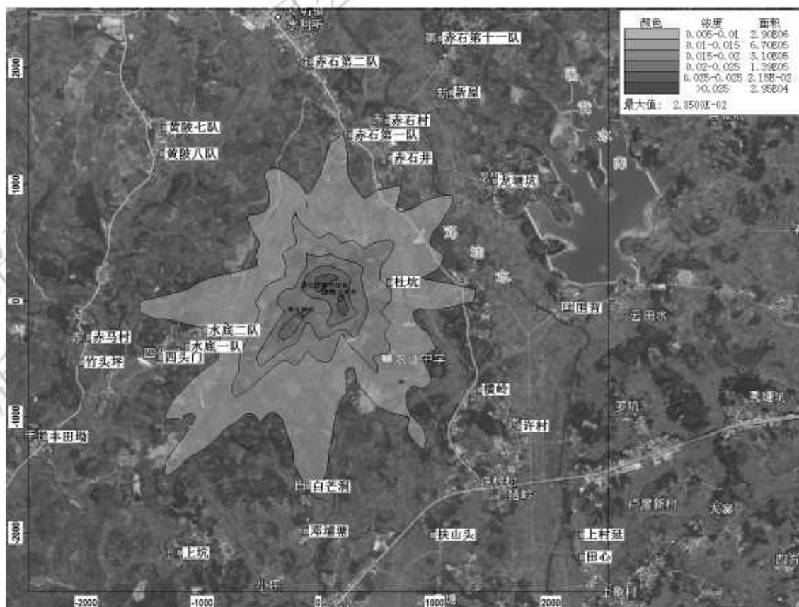
图 5-2 正常排放情况下 \text{NH}_3 小时平均浓度最大值分布图
