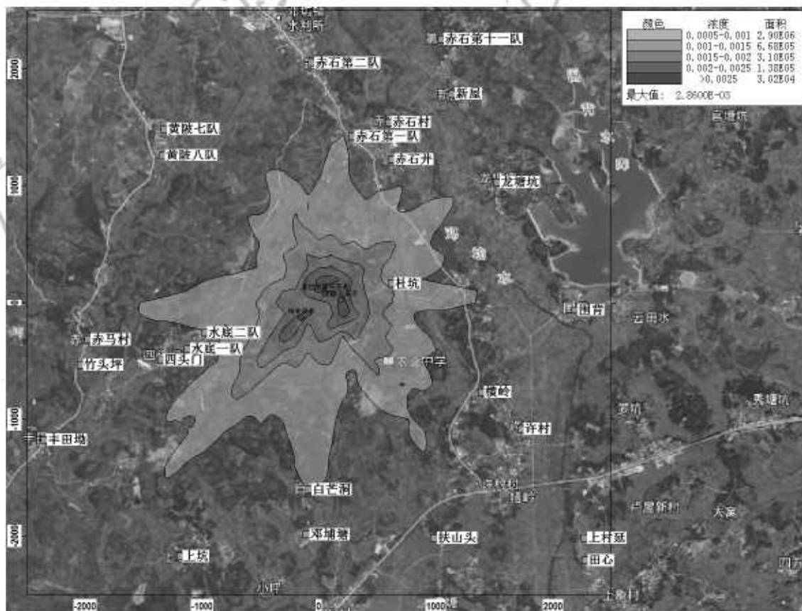
图 5-3 正常排放情况下 \text{H}_2\text{S} 小时平均浓度最大值分布图
