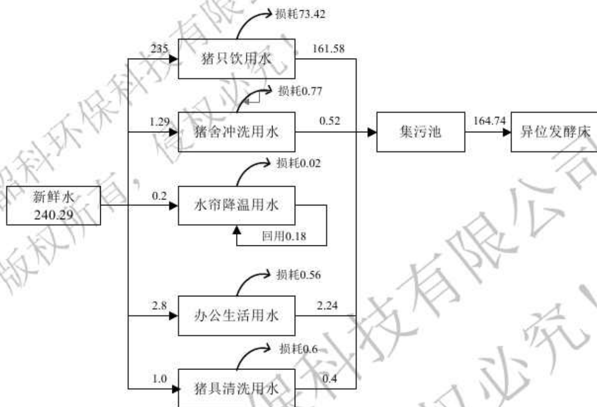
图 3-3 本项目水平衡图 (单位: m^3/d )
