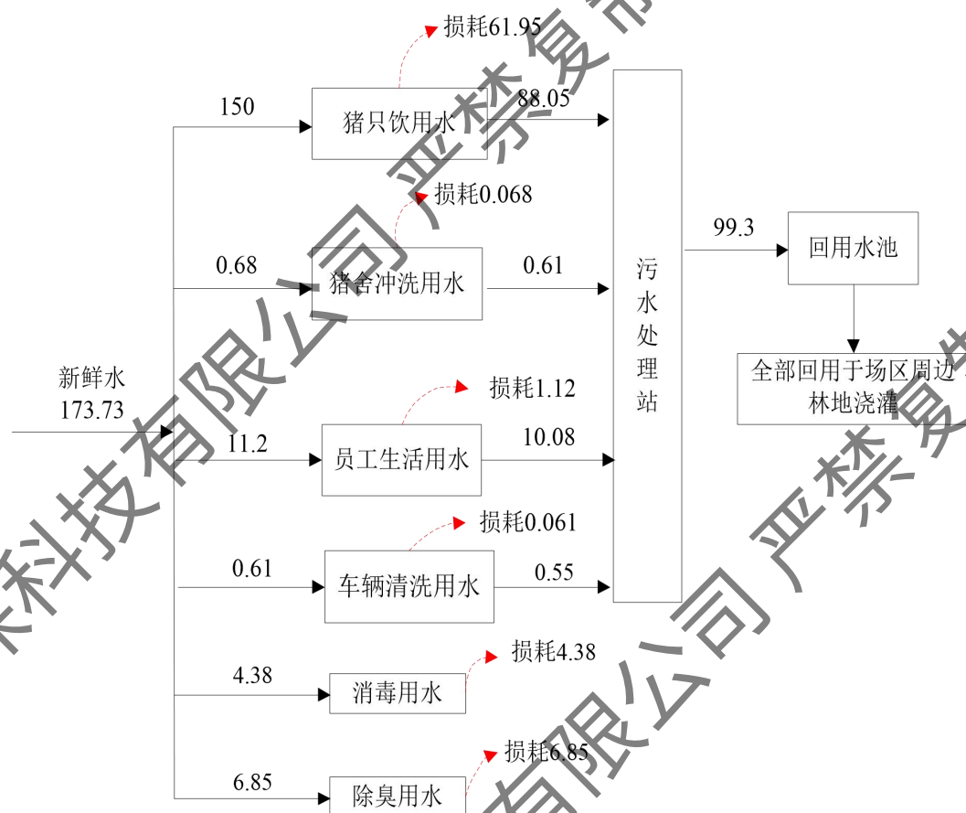
图3.2-2 项目非高温季节水平衡图 (单位: \text{m}^3/\text{d} )
