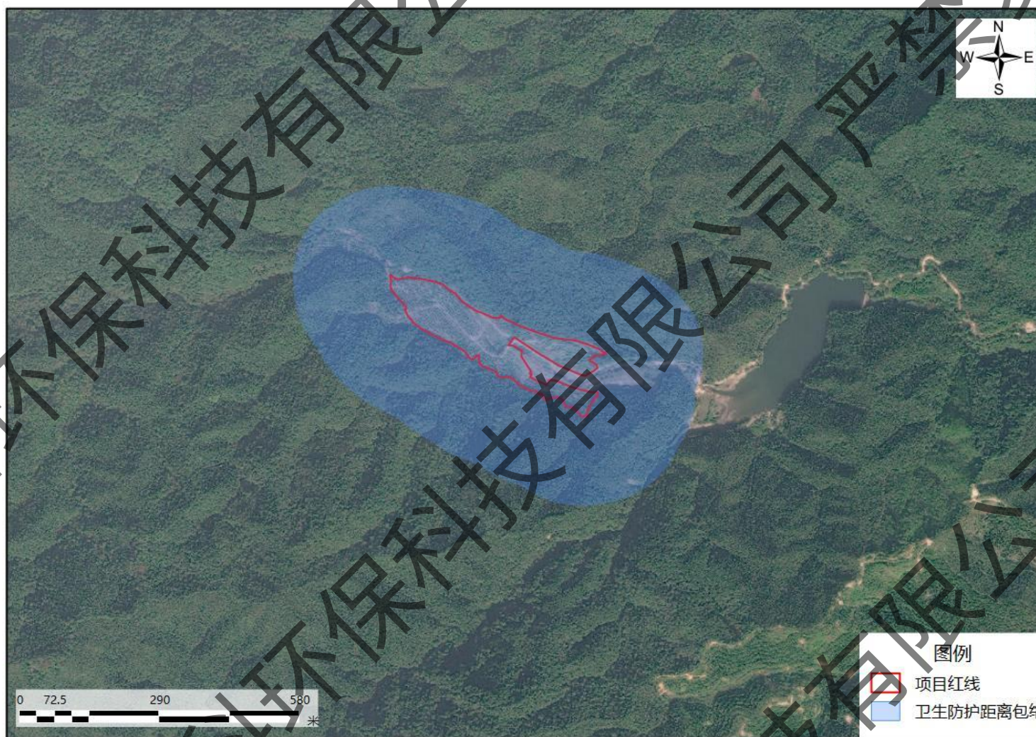
图 5.3-3 卫生防护距离包络线图
