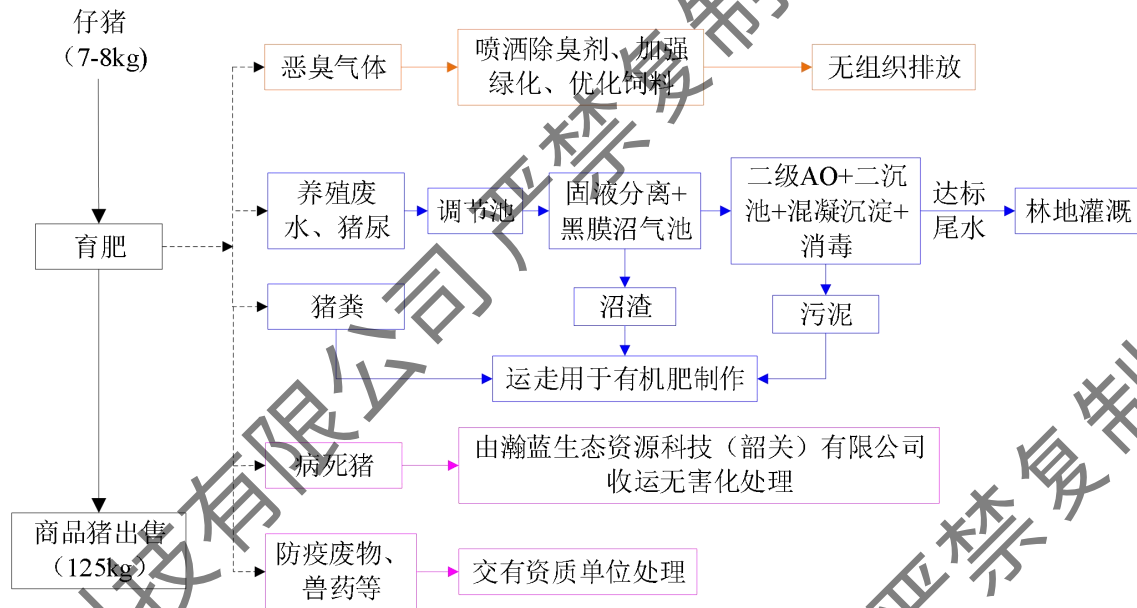
图 3.4-1 建设项目猪场饲养工艺流程图
