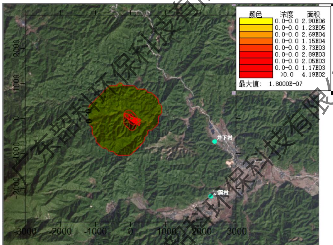
图 5.3-12 正常工况 SO 2 年均浓度贡献值分布图 (mg/m 3 )
