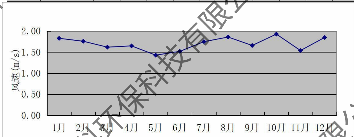
图 5.3-3 始兴气象站 2024 年各月平均风速变化图
